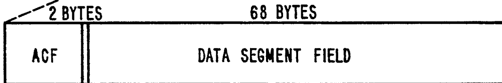
FIG. 2B SLOT FORMAT
