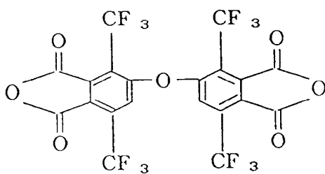
IV-(3): 2,2'-bis(fluoromethyl)-3,3',4,4'-tetracarboxydiphenyl ether anhydride
