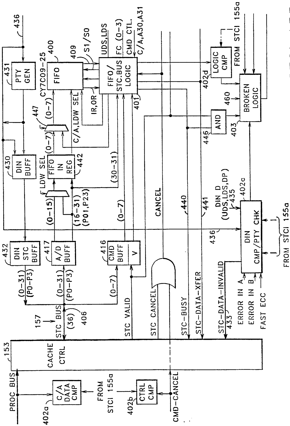
FIG. 32A - STCI 155
