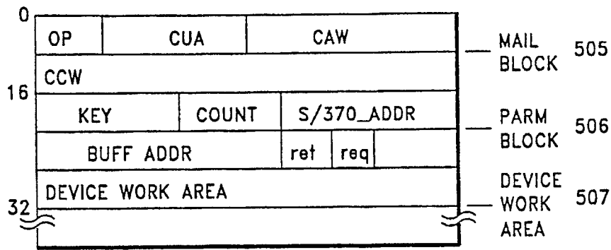
FIG. 41D - WQB
