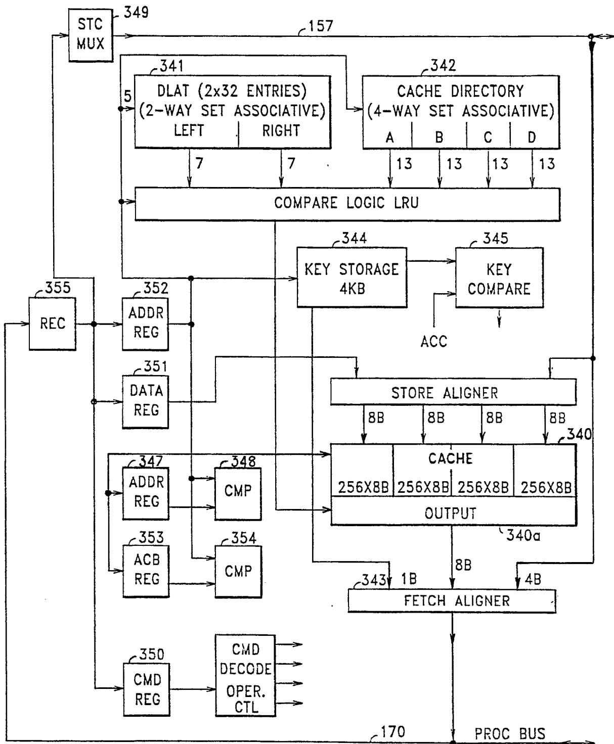
FIG. 31 - CACHE CONTROLLER 153
