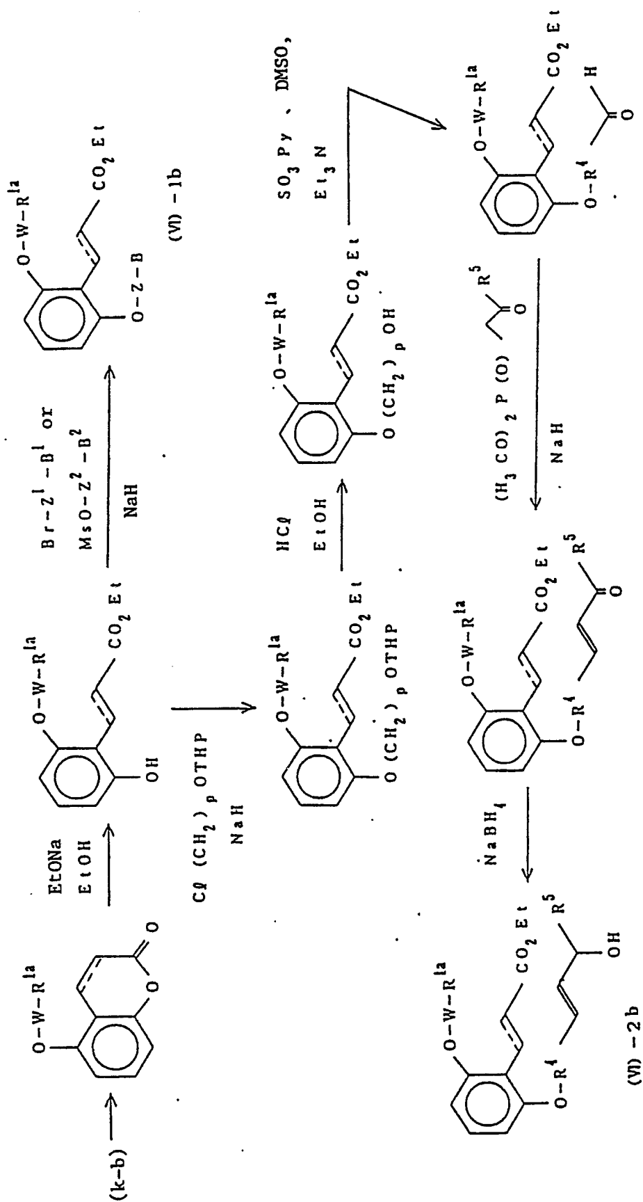
Scheme [C]-1b (cont'd)
