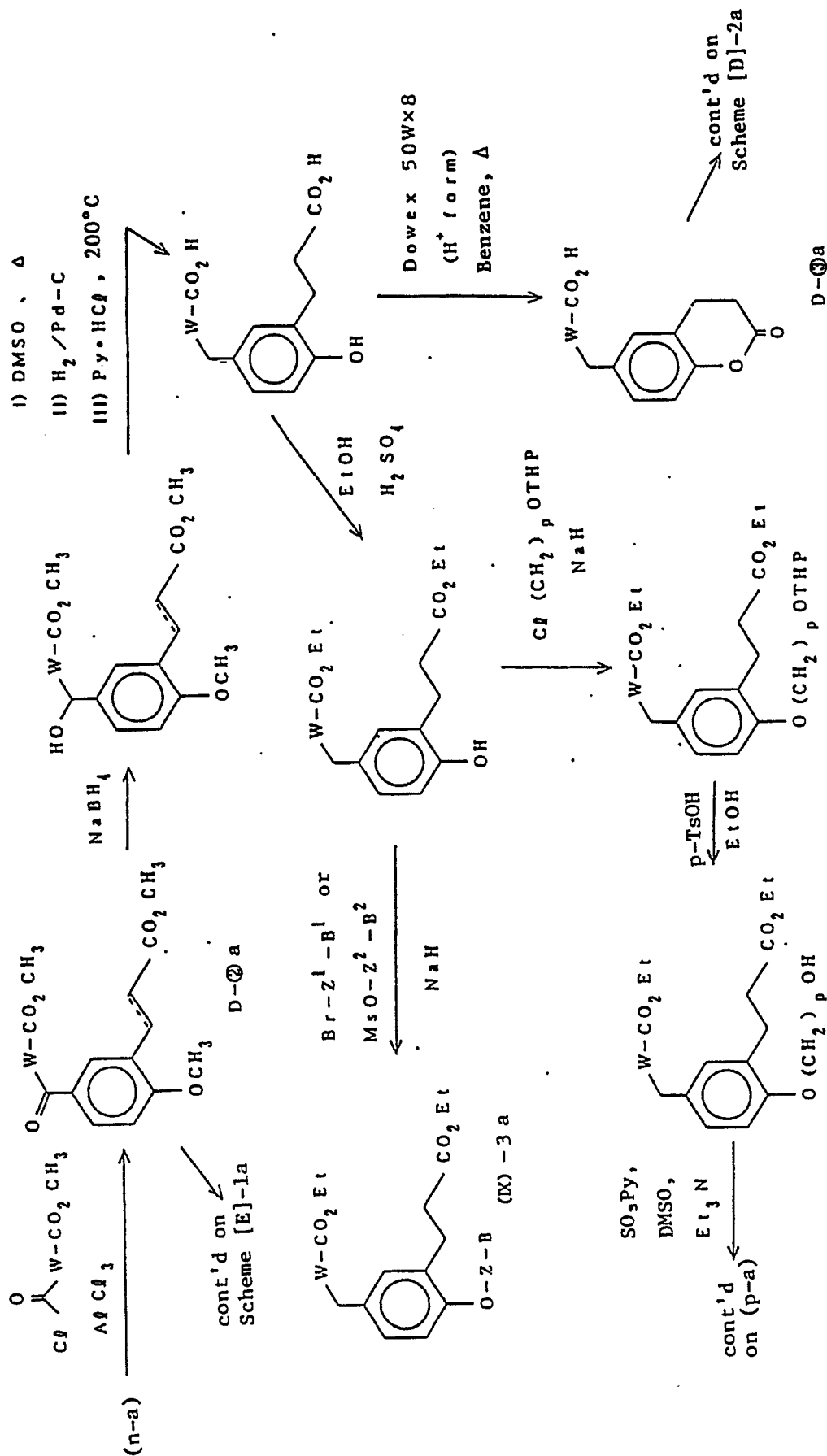
Scheme [D]-1a (cont'd)
