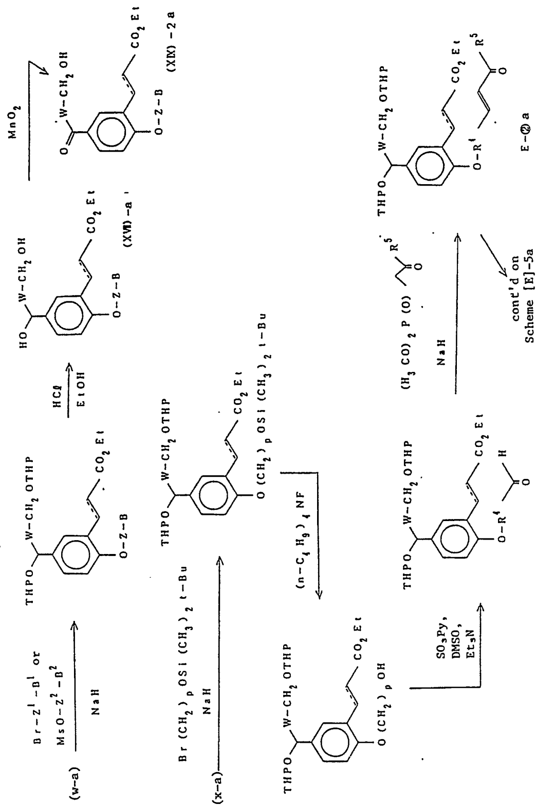
Scheme [E]-4a (cont'd)
