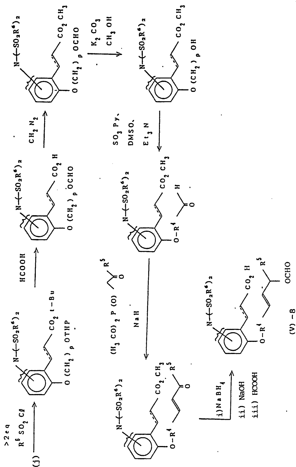
Scheme [B]-3 (cont'd)
