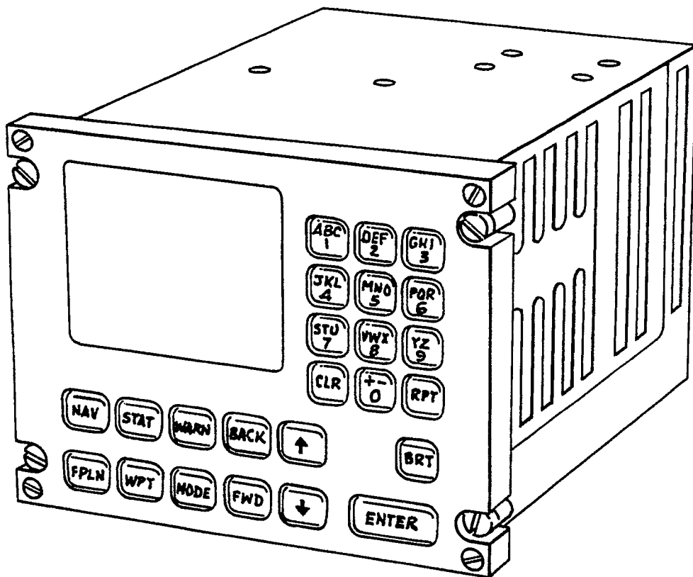
FIG. 11. THE CDU.
