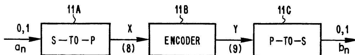
FIG. 2B
