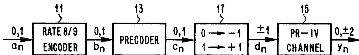
FIG. 2A
