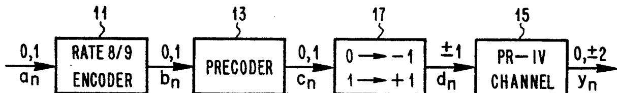
FIG. 2A
