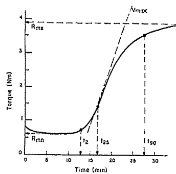
VULCANIZATION PARAMETERS
