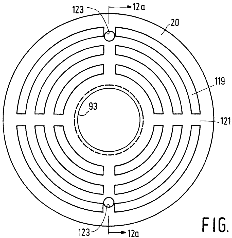
FIG.12a
