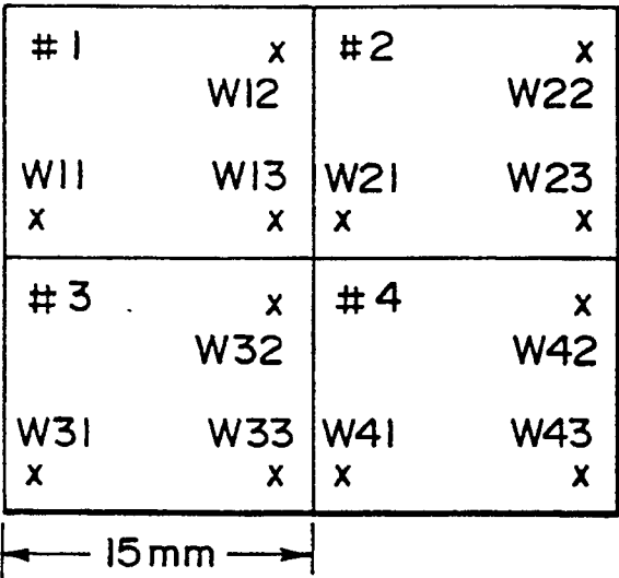
FIG. 15A WAER PATTERN
