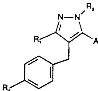
Formule (I)
