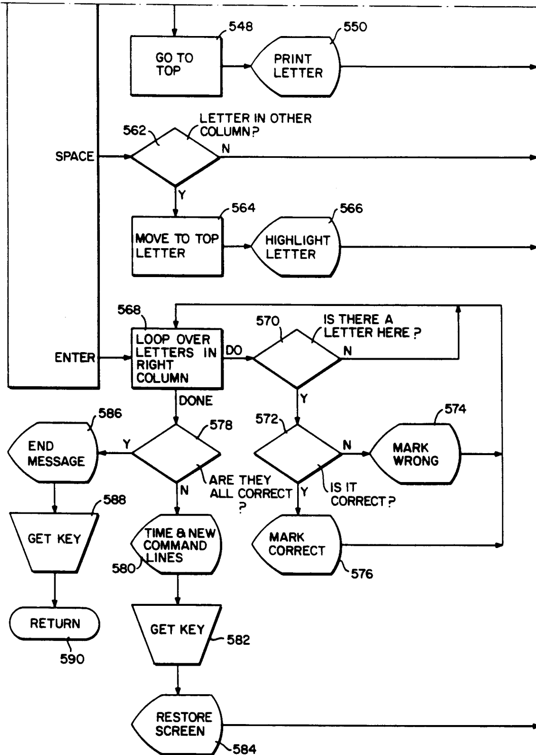
FIG. 9E "SOUND SORT" ROUTINE
