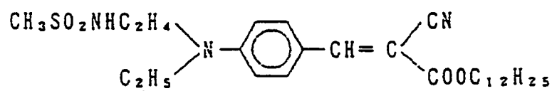
C p d - 6
