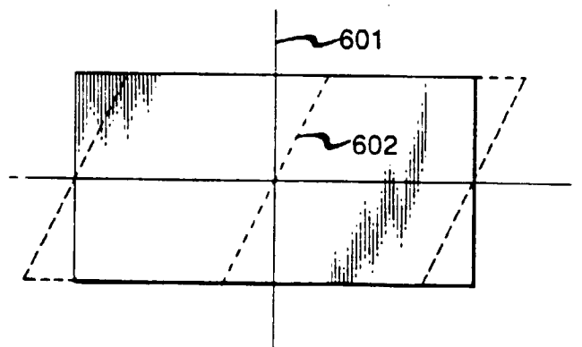
FIG. 6 \gamma_{XY} : SHEAR
