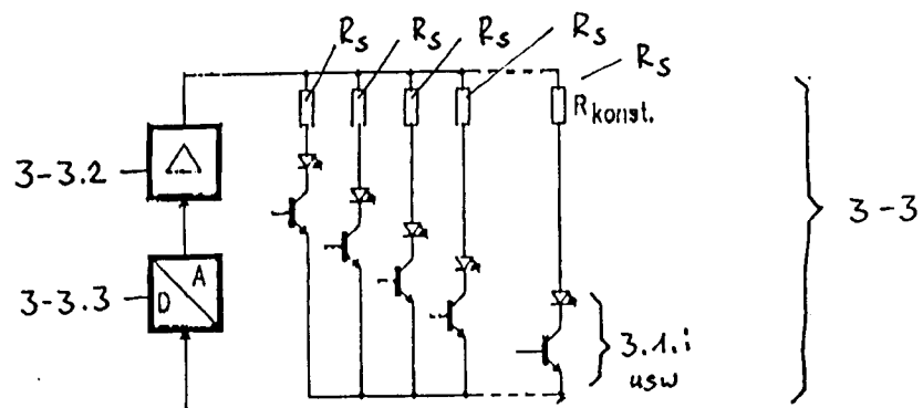
Blockschema Steuerung des Sendestroms durch Steuerung der Spannung und konstantem Vorwiderstand
