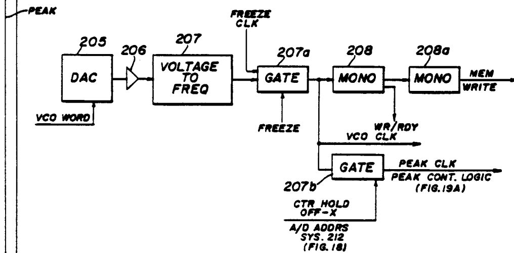
FIG. 18D VCO CLOCK GEN. 204
