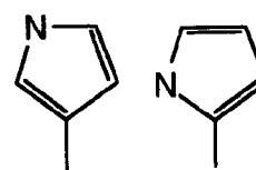
Pyrroles
