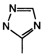
Triazoles
