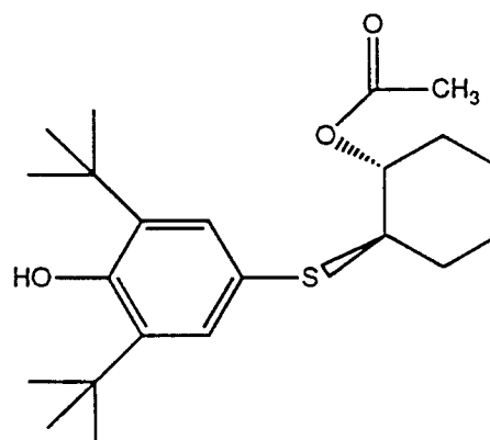
(-) ISOMER R,R
