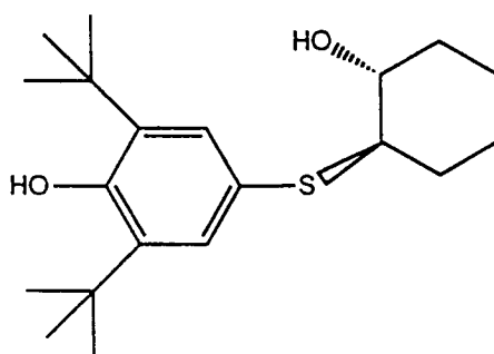
(-) ISOMER R,R
