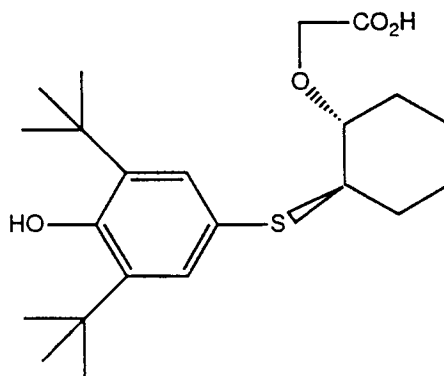
(-) ISOMER R,R
