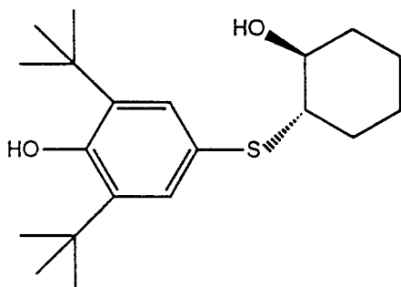
(+) ISOMER S,S
