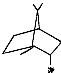
born-2-yl
