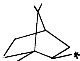
isoborn-2-yl
