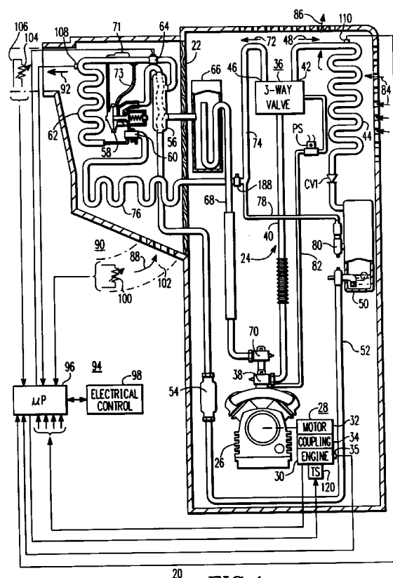
20 FIG.1
