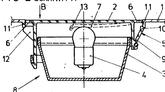
FIG 2 Schnitt A-A
