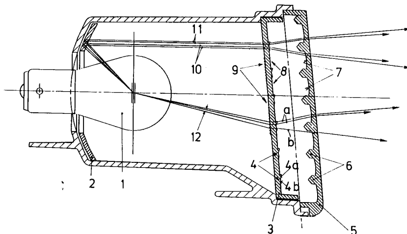
FIG 2 Schnitt A-A
