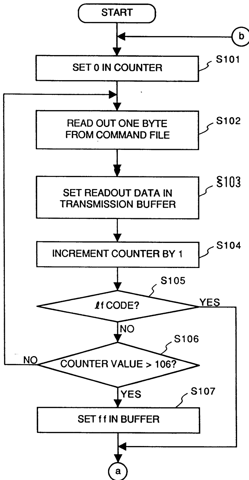
FIG. 23A
