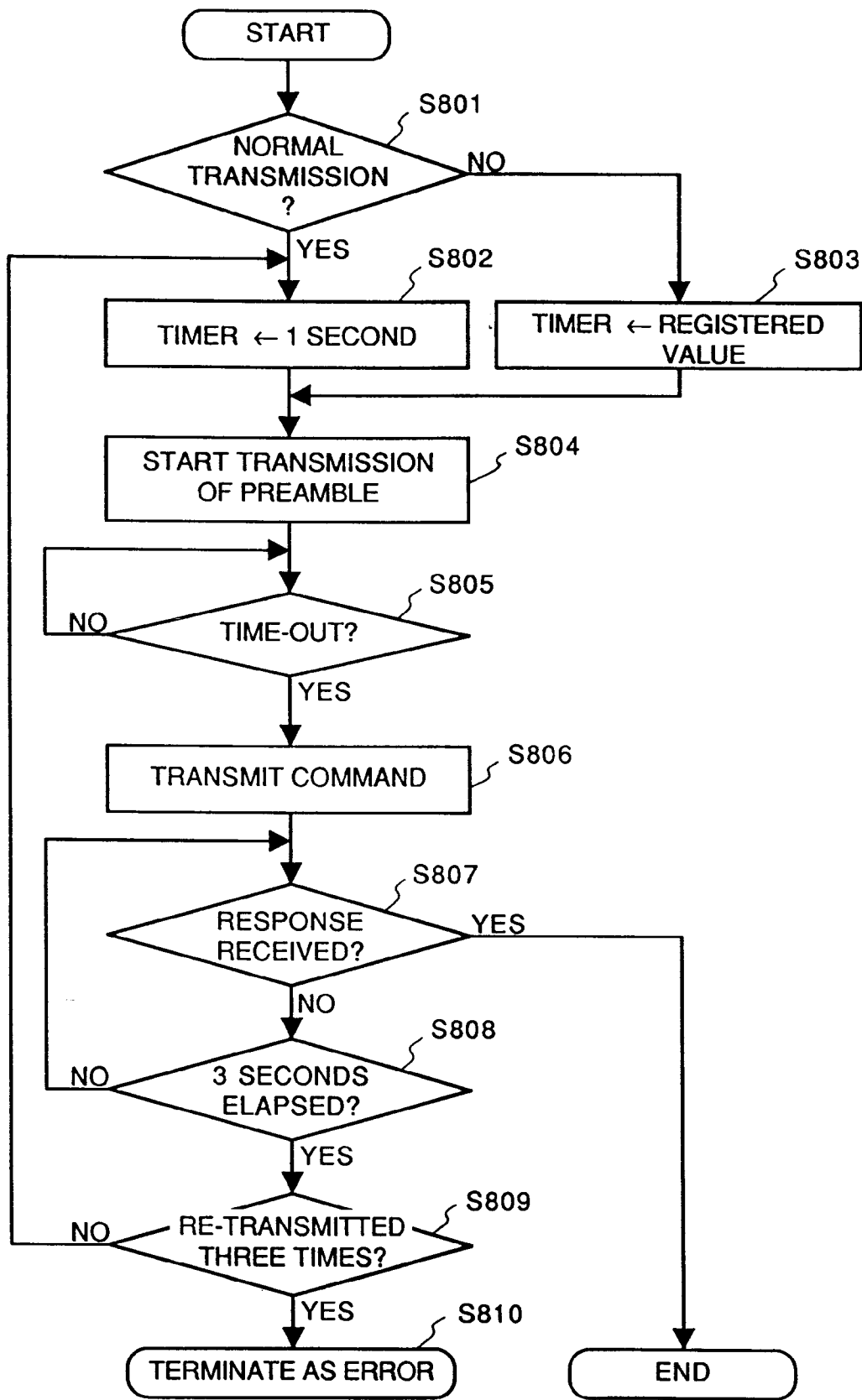
FIG. 50
