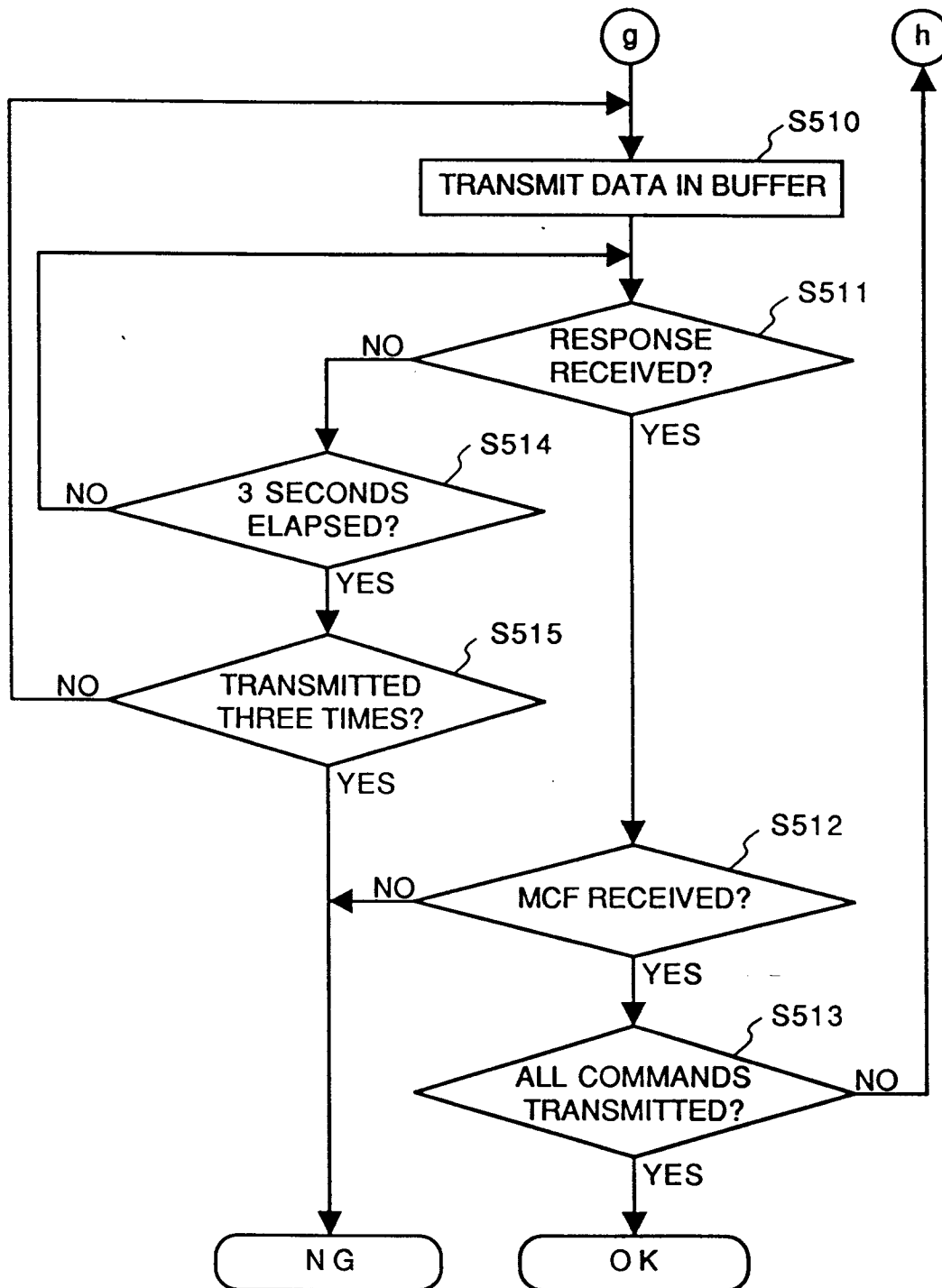
FIG. 30B
