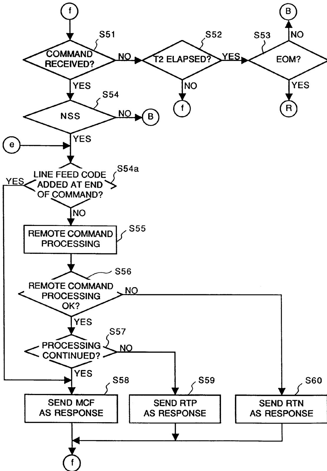
FIG. 9A
