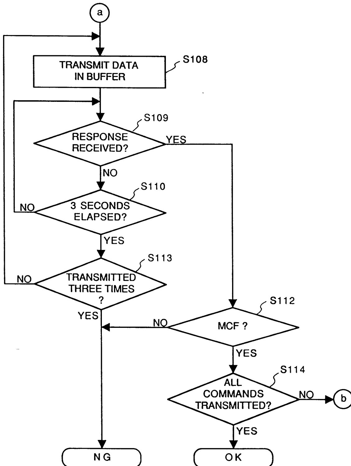
FIG. 23B
