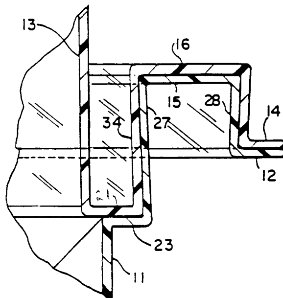
FIG. 8 (ENLARGED DETAIL)
