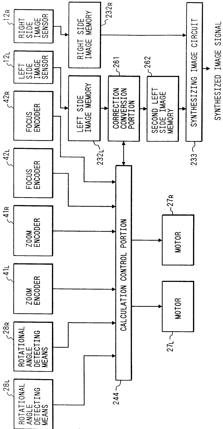
FIG. 26B
