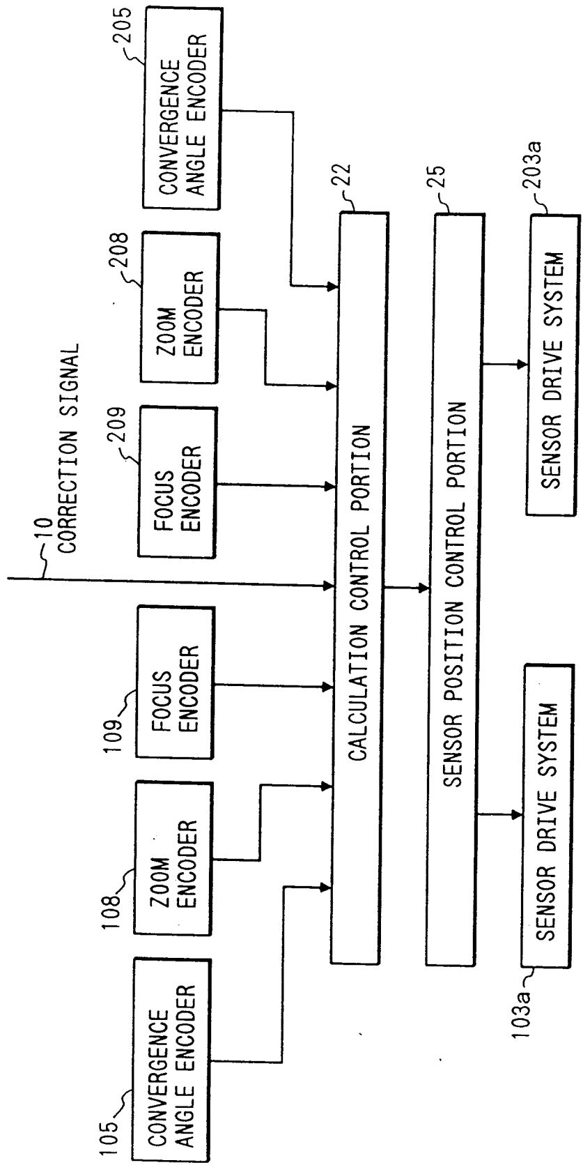
FIG. 38
