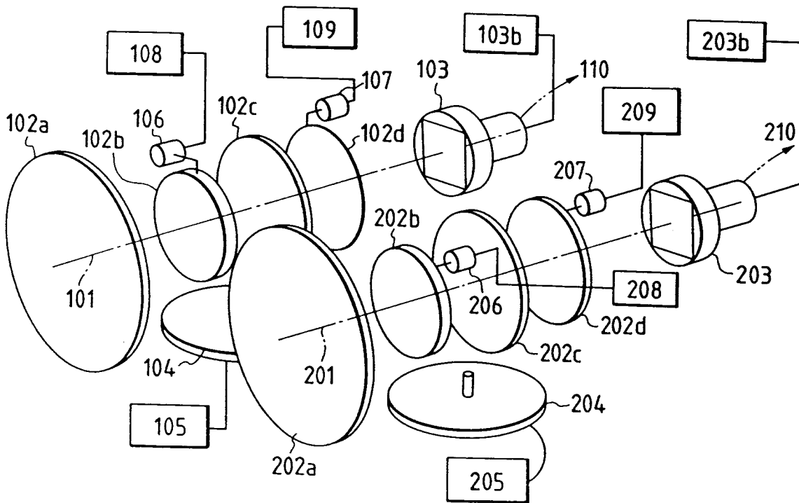
FIG. 39
