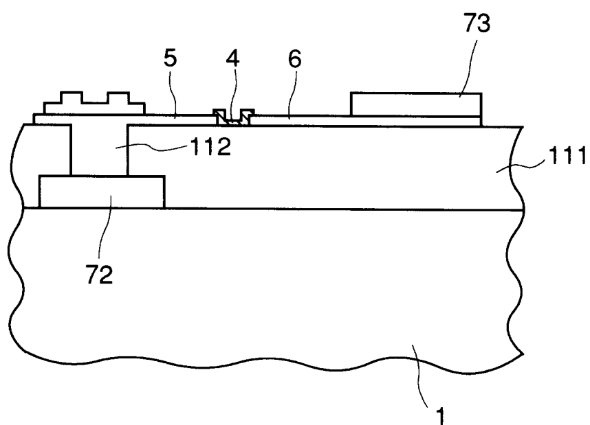
A-A' SECTION
