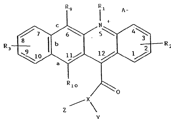
Formula II: LBAC
