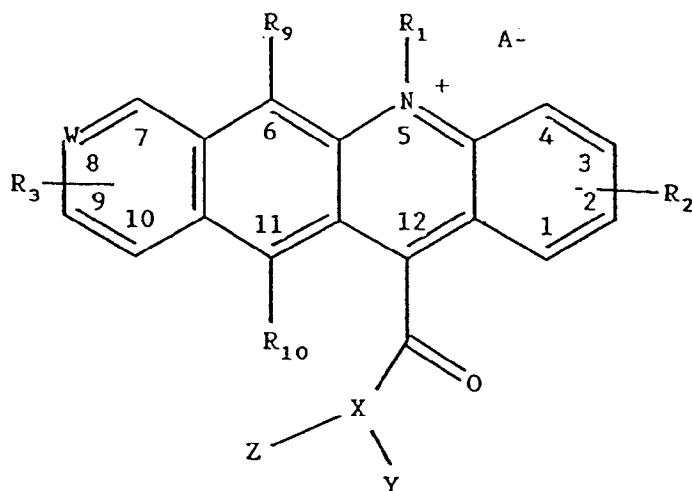
Formula I: AFAC
