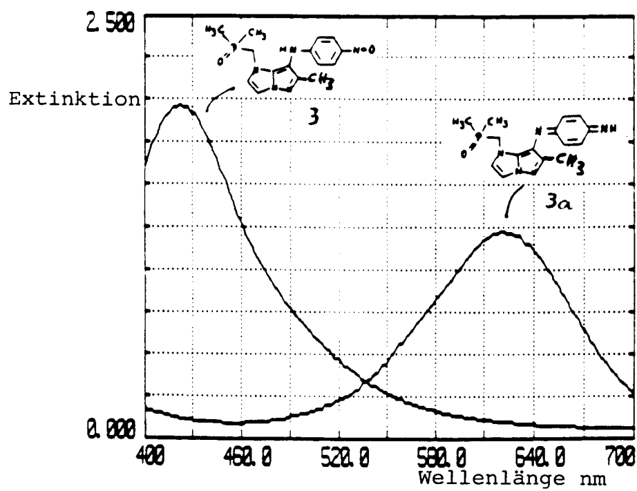
Fig. 5: Spektren von p-Nitrosoanilin (3) und Chinondiimin (3a)
