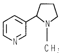
nicotine
