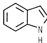
indole
