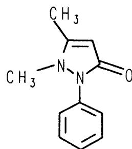
antipyrine
