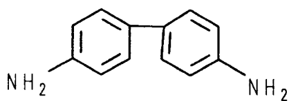
benzidine
