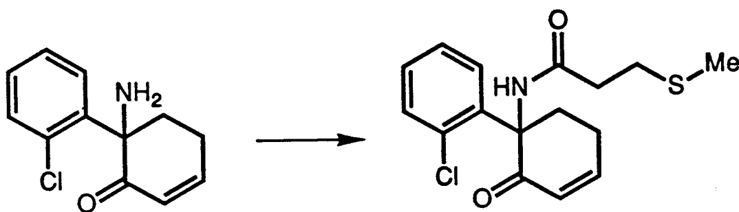
6-(2-Chlorophenyl)-6-(3-(methylthio)propanoyl)amino-2-cyclohexen-1-one
