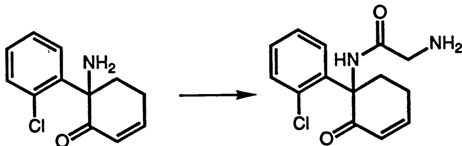
6-(2-Aminoacetyl)amino-6-(2-chlorophenyl)-2-cyclohexen-1-one
