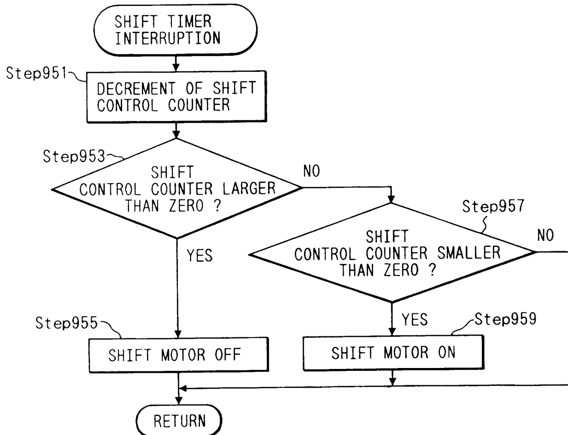
FIG. 30B
