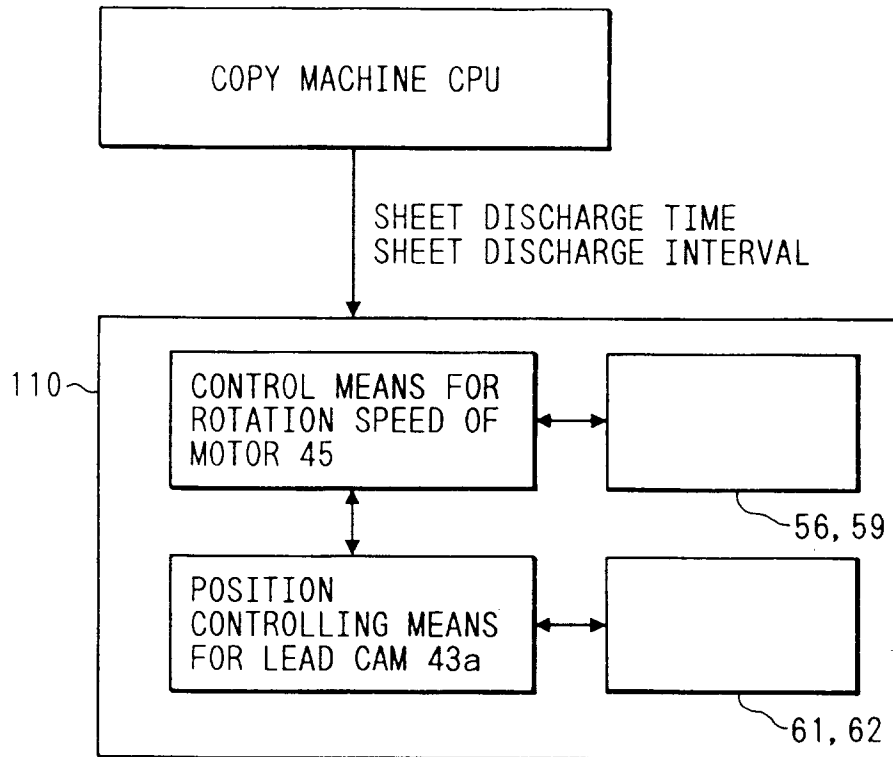
FIG. 31
