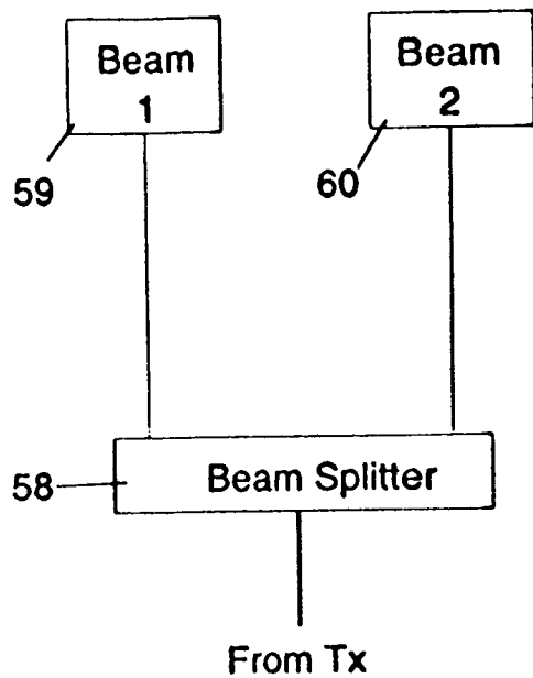
Fig. 14 (a) Inphase
