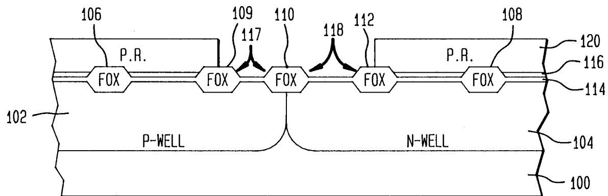
FIG. 5C
