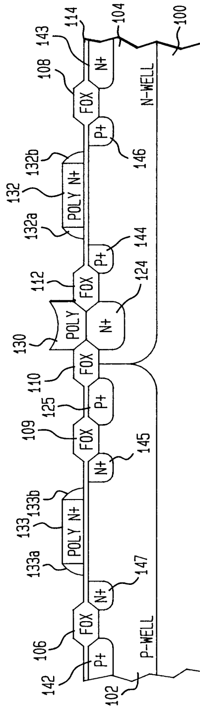
FIG. 2E
