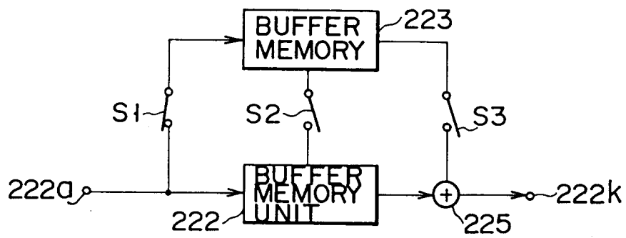
F I G. 29A
