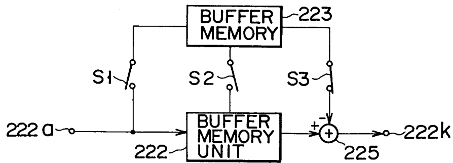
F I G. 29A
