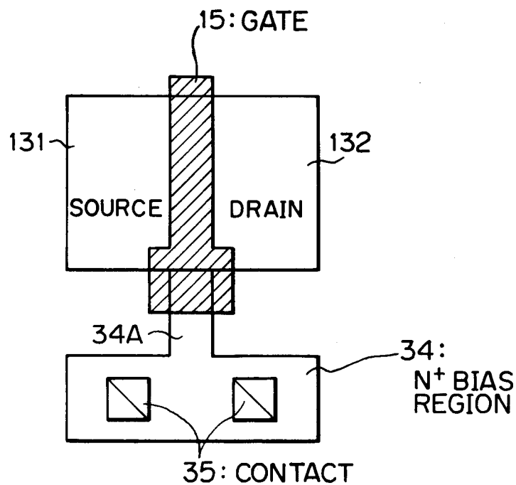
SOI MOSFET
