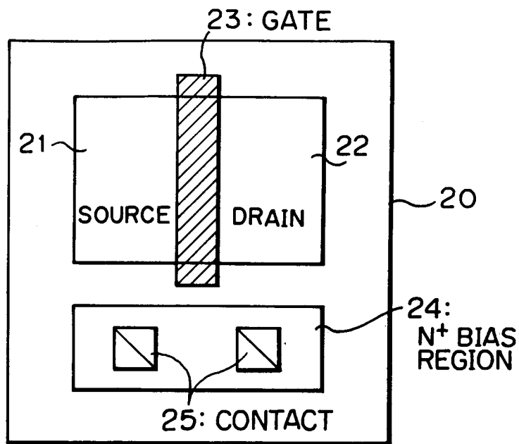
BULK MOSFET
