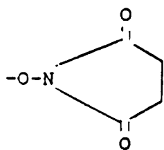
Oxysuccinimide
