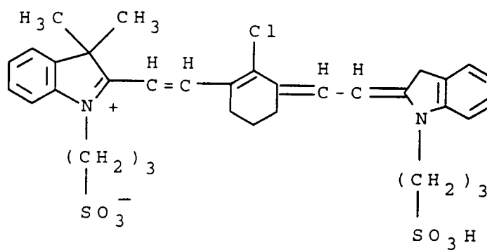
IR-3 IR-Absorbing Dye
