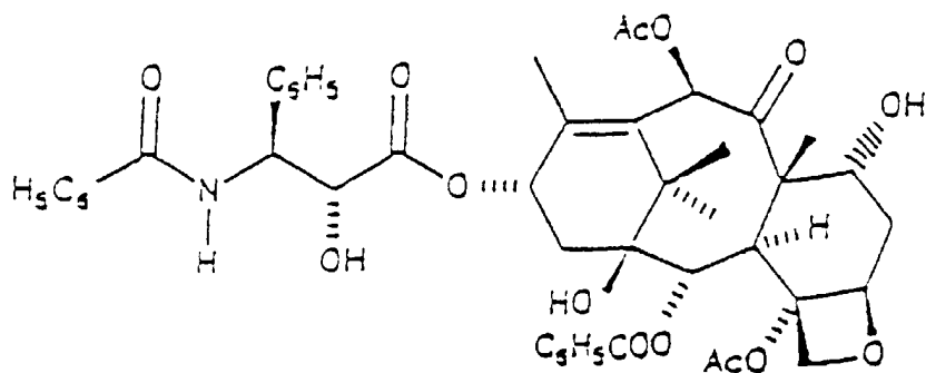
7-EPITAXOL
