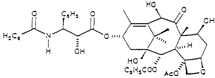
10-DESACETYLTAXOL
