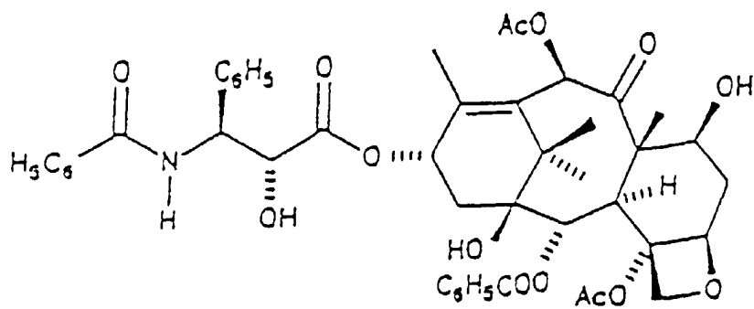
TAXOL
