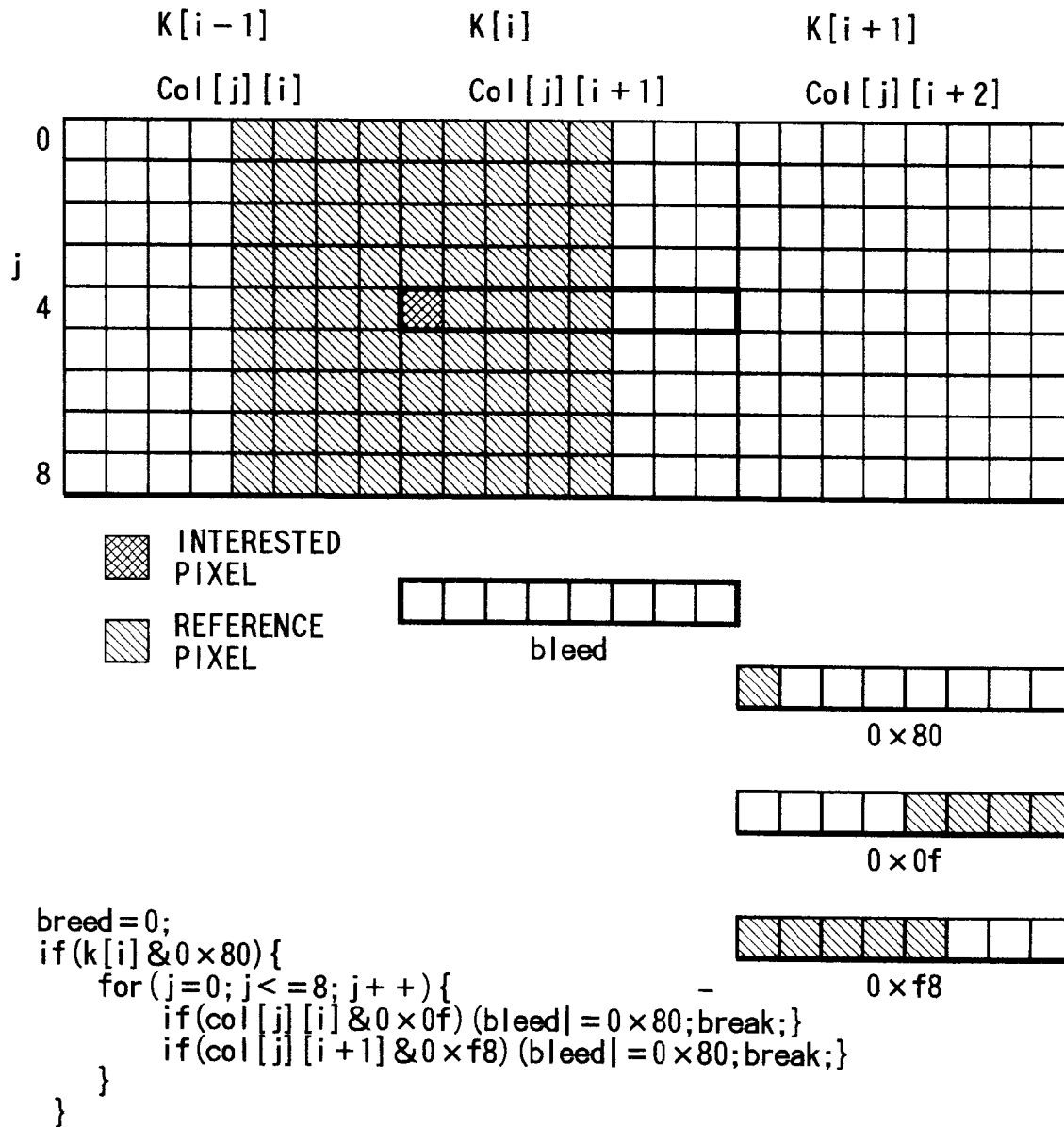
FIG. 63
