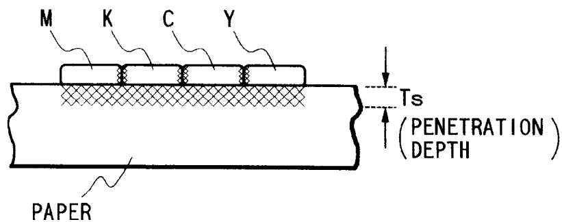
FIG. 53B
