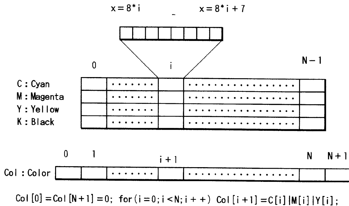
FIG. 62
