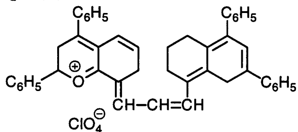
Dye (d)
