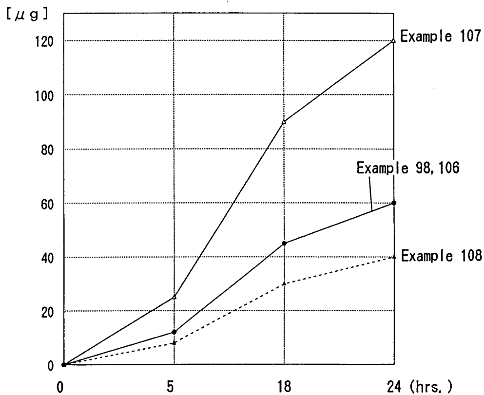
Fig. 3 1 Permeation Test (17- \beta -estradiol)
