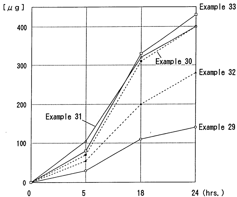
Fig. 1 3 Permeation Test (17- \beta -estradiol)
