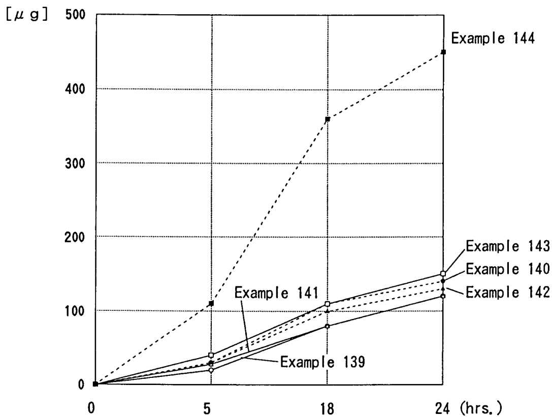
Fig. 5 9 Permeation Test (17- \beta -estradiol)
