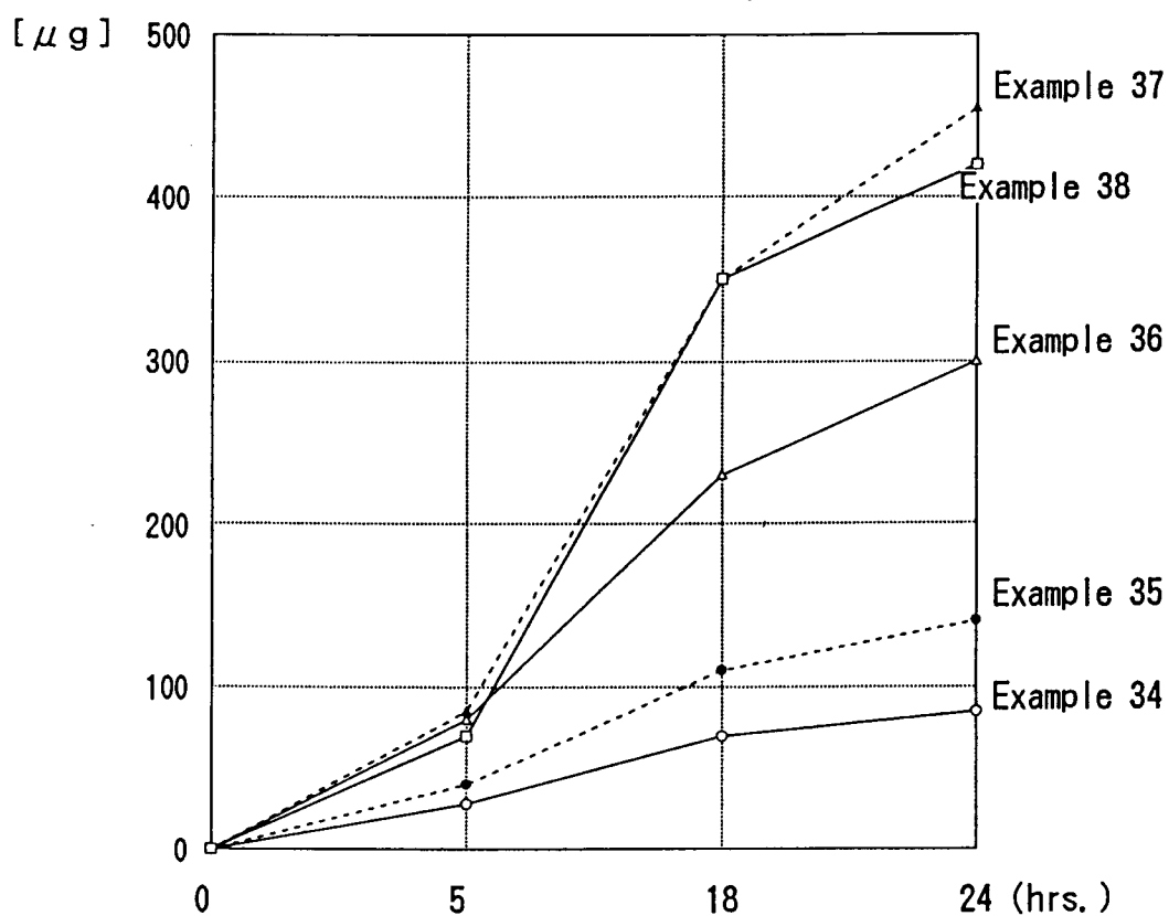
Fig. 1 5 Permeation Test (17- \beta -estradiol)
