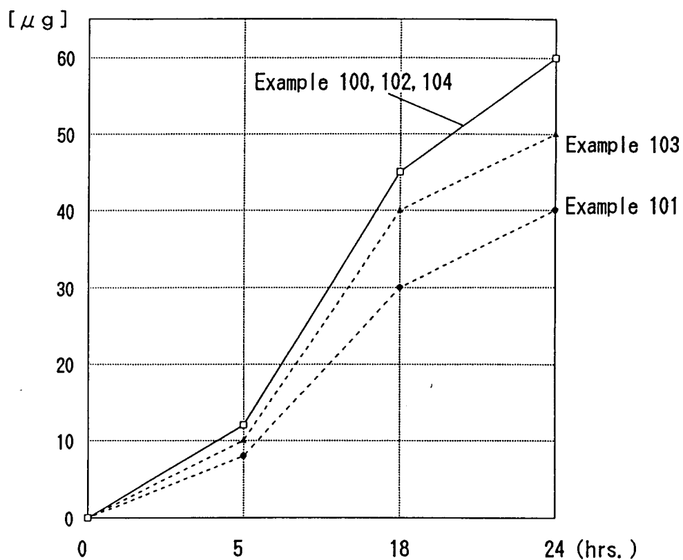
Fig. 3 0 Permeation Test (17- \beta -estradiol)
