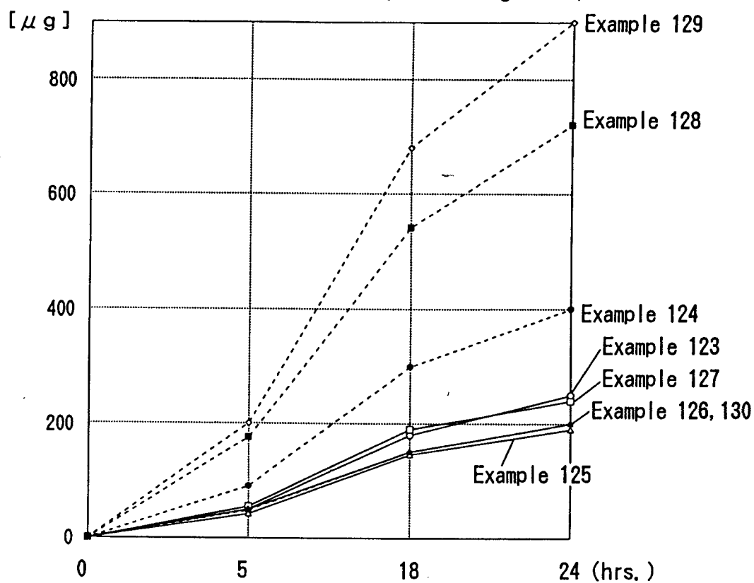
Fig. 5 4 Permeation Test (3-ketodesogestrel)
