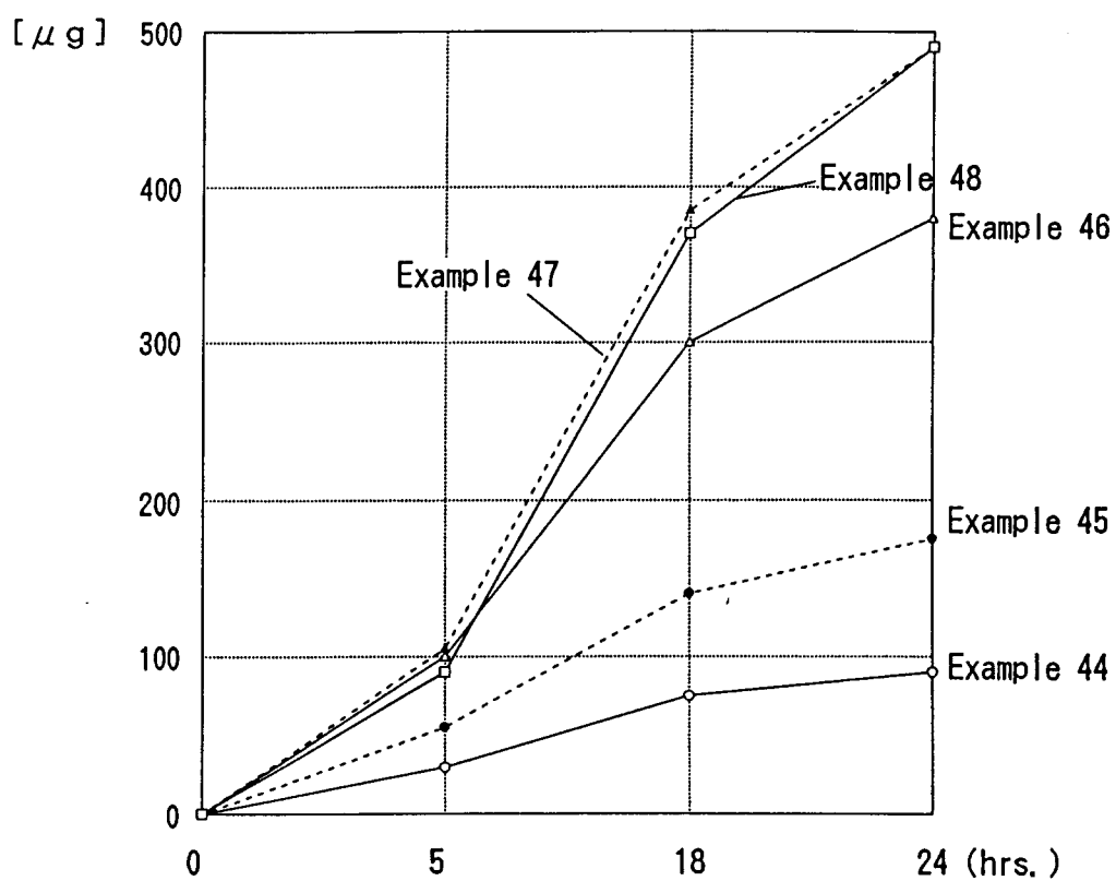
Fig. 1 9 Permeation Test (17- \beta -estradiol)
