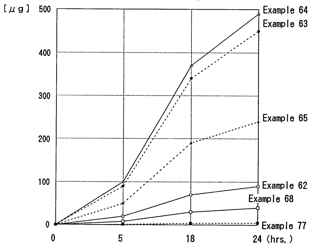
Fig. 2 5 Permeation Test (17- \beta -estradiol)
