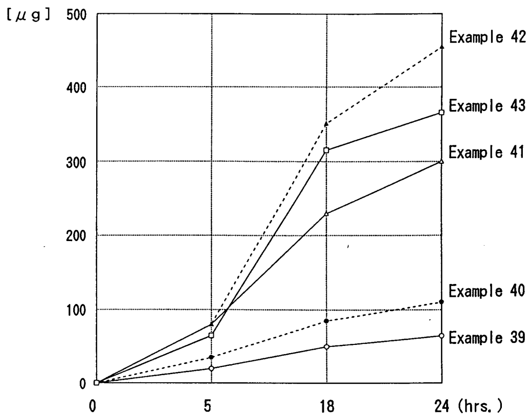
Fig. 1 7 Permeation Test (17- \beta -estradiol)
