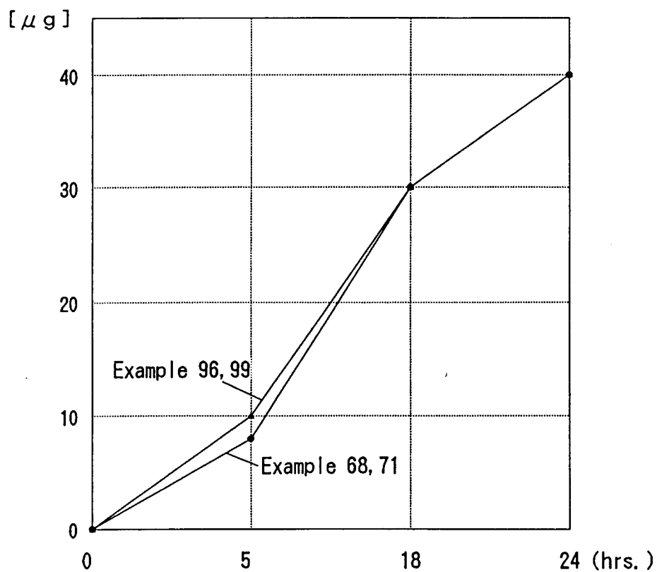
Fig. 4 8 Permeation Test (17- \beta -estradiol)
