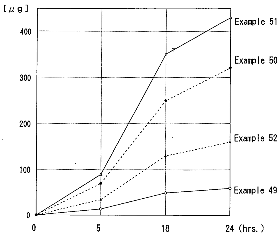
Fig. 2 2 Permeation Test (17- \beta -estradiol)
