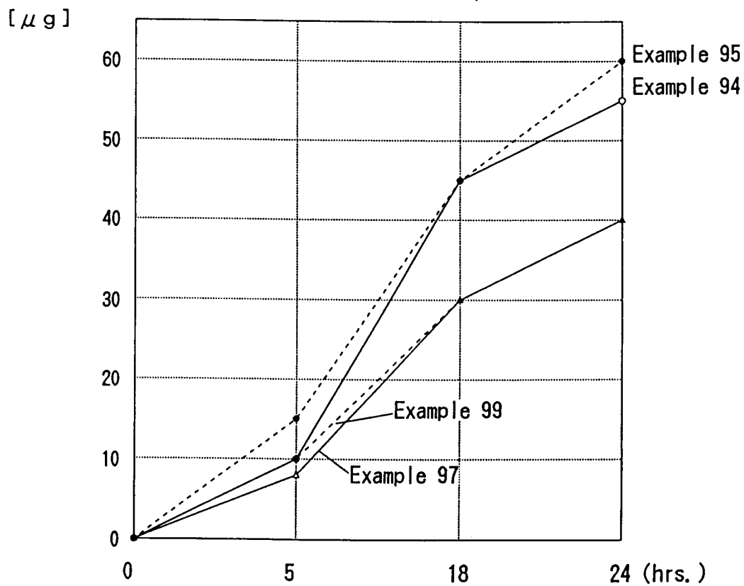
Fig. 2 9 Permeation Test (17- \beta -estradiol)
