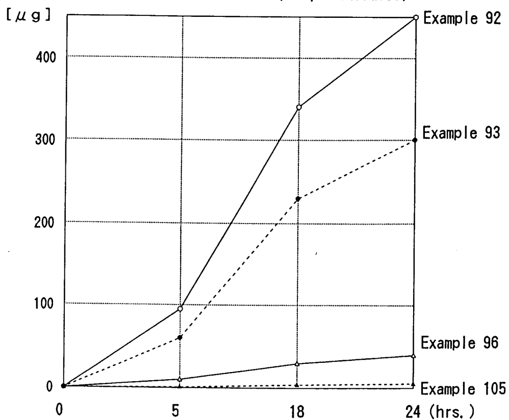
Fig. 2 8 Permeation Test (17- \beta -estradiol)
