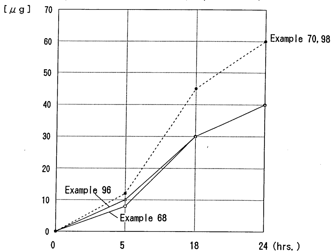
Fig. 5 0 Permeation Test (17- \beta -estradiol)
