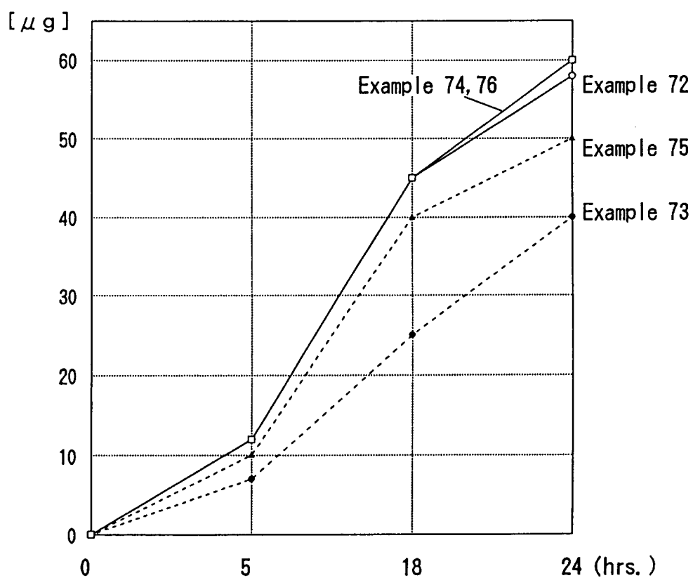
Fig. 2 7 Permeation Test (17- \beta -estradiol)
