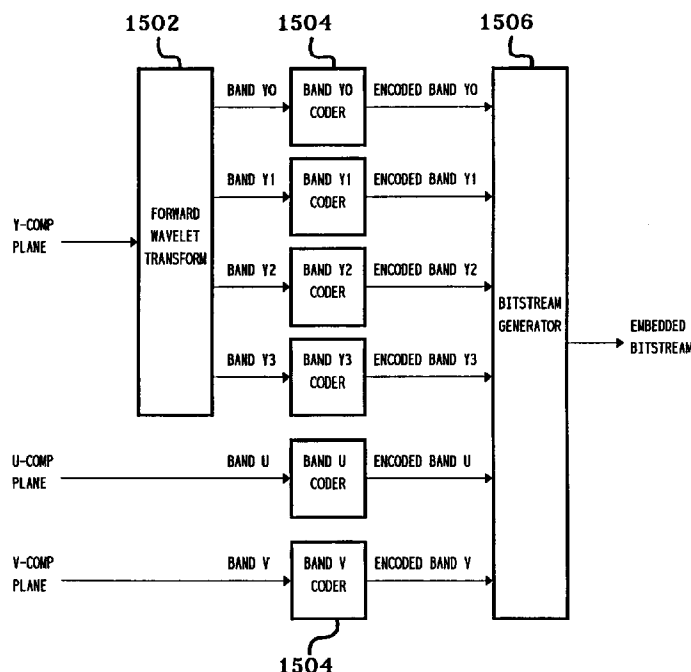
FIG. 15. ENCODER
