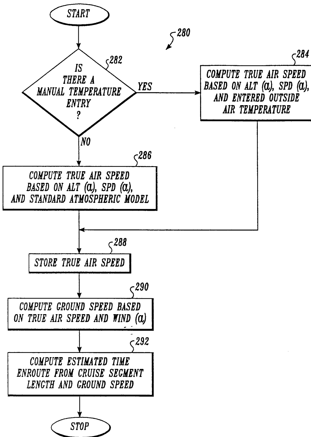
FIG. 4G.
