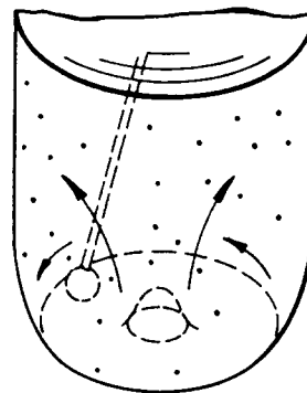
c) Neuentwickelte Kulturflasche für Microcarrierkulturen. Die Anordnung des kugelförmigen Magneten in der kreisförmigen Bodenrinne ermöglicht höhere Zellausbeuten als bei herkömmlichen Spinnergefäßen
