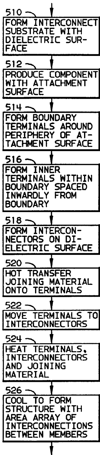
FIG. 16
