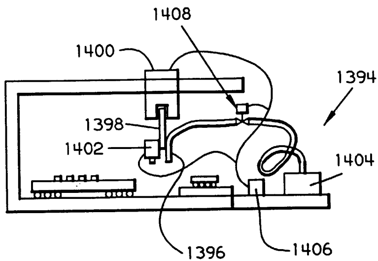
FIG. 74(h)
