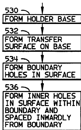
FIG. 17
