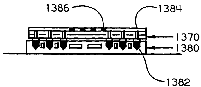
FIG. 74 (f)
