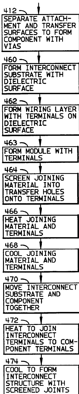
FIG. 14
