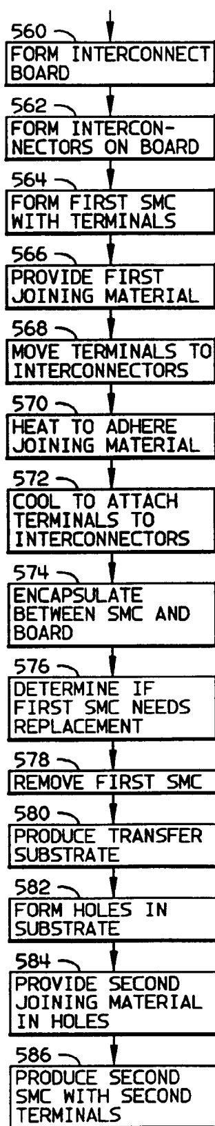
FIG. 20(a)
