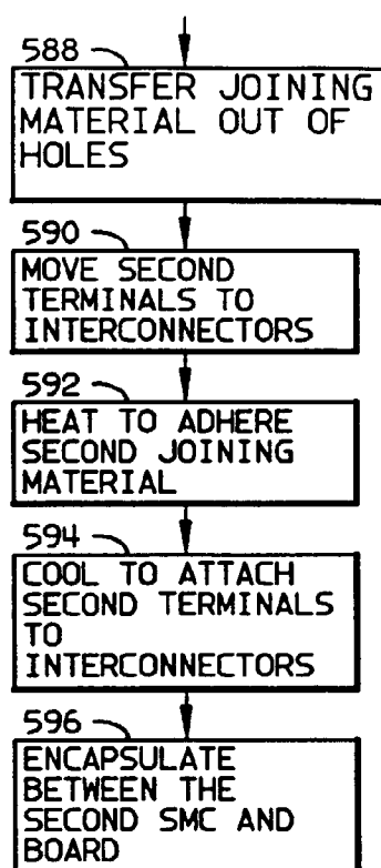
FIG. 20(b)
