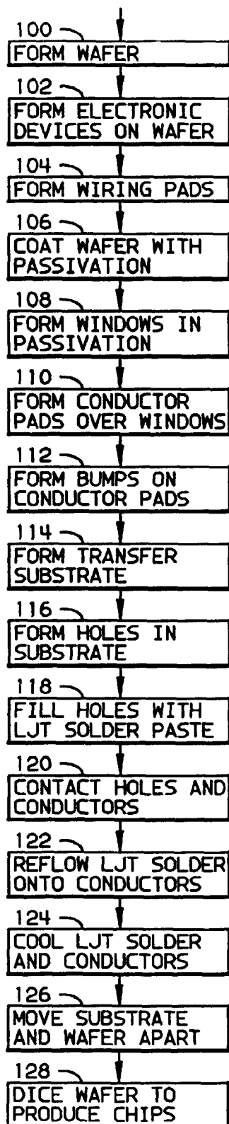
FIG. 1
