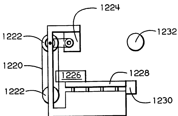
FIG. 73 (b)
