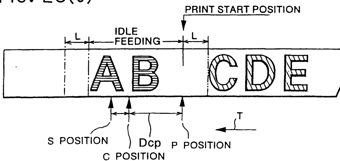
FIG. 28(c)
