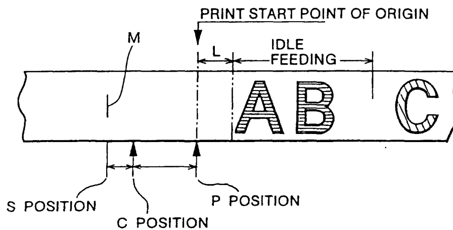
FIG. 35(b)
