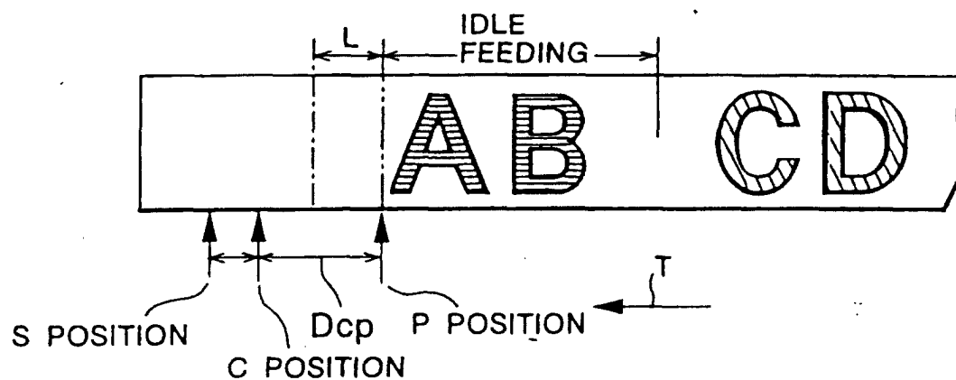
FIG. 28(c)
