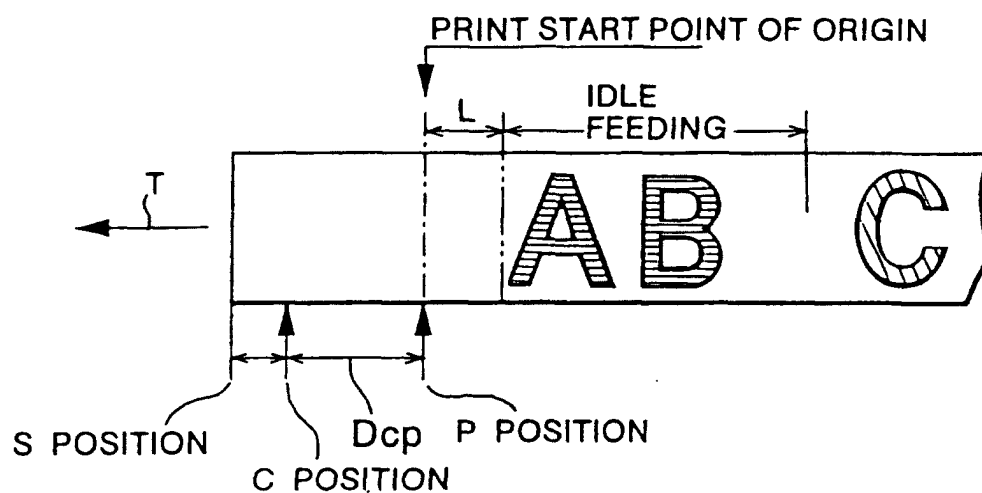
FIG. 28(b)
