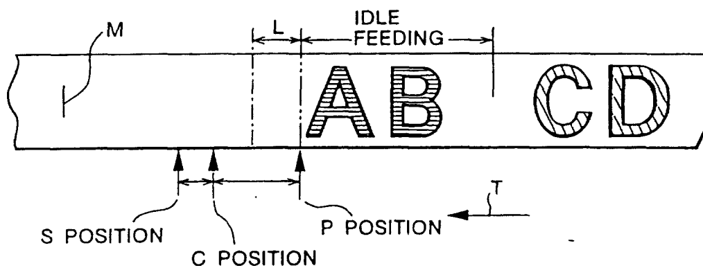
FIG. 35(c)
