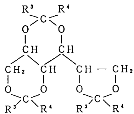
(IIIb)
