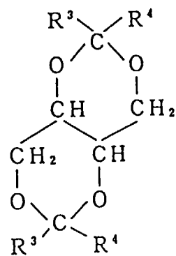
(IVb)
