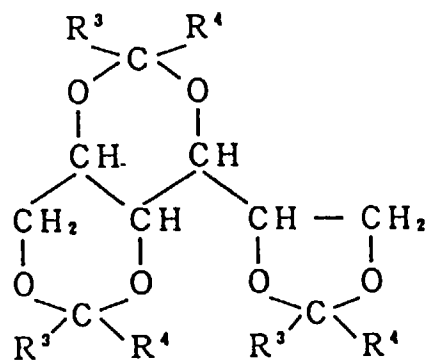
(IIIb)
