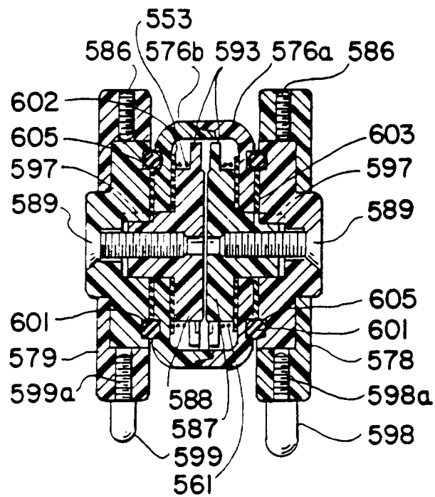
FIG. 49
