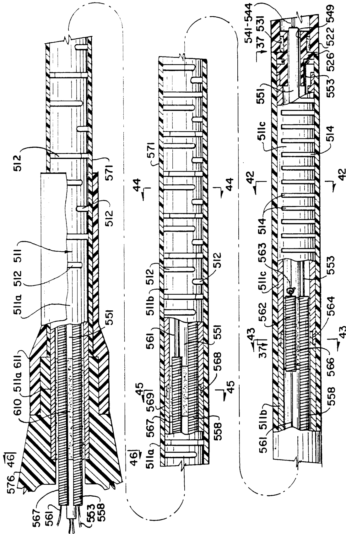
FIG. 36
