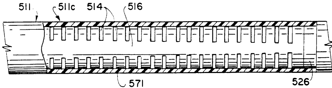
FIG. 37
