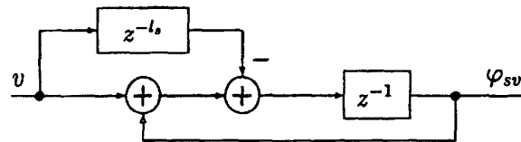
Fig. 12: Korrelationsfilter für den Horizontal-Synchronimpuls
