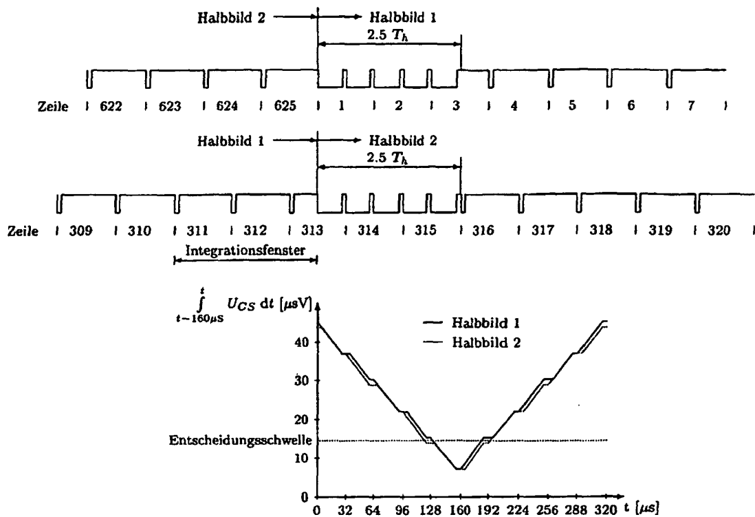
Fig. 4: Vertikal-Synchronsignal und seine Aufintegration über 160 \mu s mit ungleichen Flanken in Abhängigkeit von der Halbbildnummer
