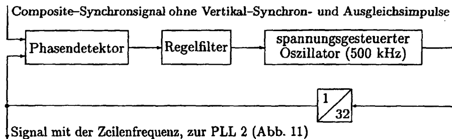
Fig. 9: Gewinnung des Composite-Synchronsignales
