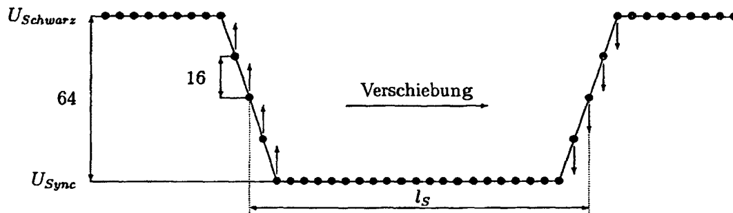
Fig. 13: Verschiebung eines Impulses um einen Bruchteil eines Pixels ( l_s = 25 )
