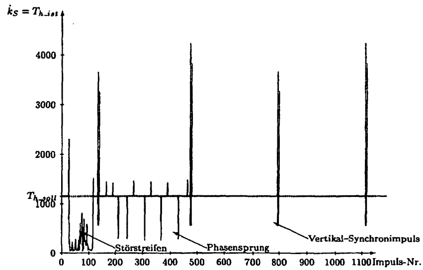
Fig. 17: Zeilenperiodendauerfolge T_{hist} = k_S am Ausgang des Synchronsignaldetektors
