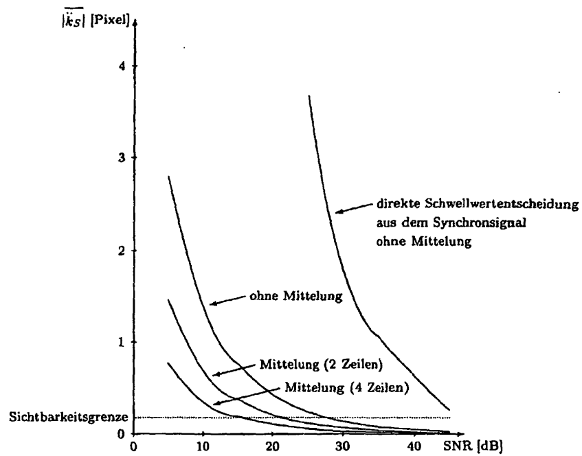
Fig. 18: mittleres Phasenrauschen bei der Synchronimpulsdetektion durch Korrelation in Abhängigkeit vom SNR des Synchronsignales
