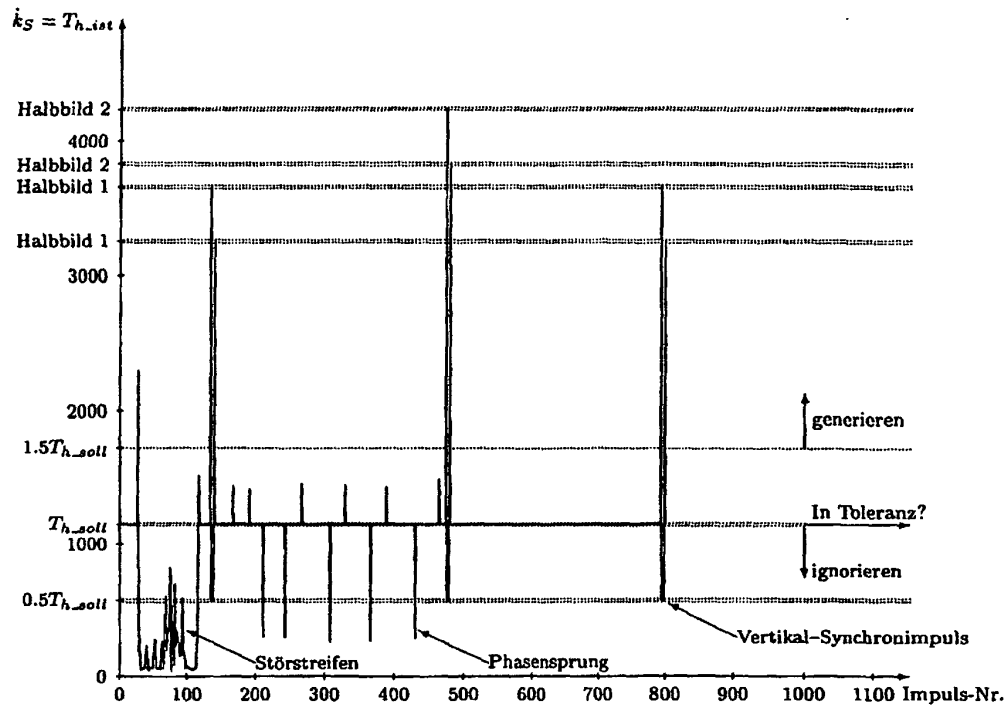
Fig. 19: Weiterverarbeitung der Zeilenperiodendauerfolge T_{h\_ist} = k_S im Horizontal-Synchronsignalgenerator und Ausnutzung der Phasen- und Frequenzmodulation der Synchronimpulse zur Vertikal-Synchronisation (siehe Abschnitt 5.4)
