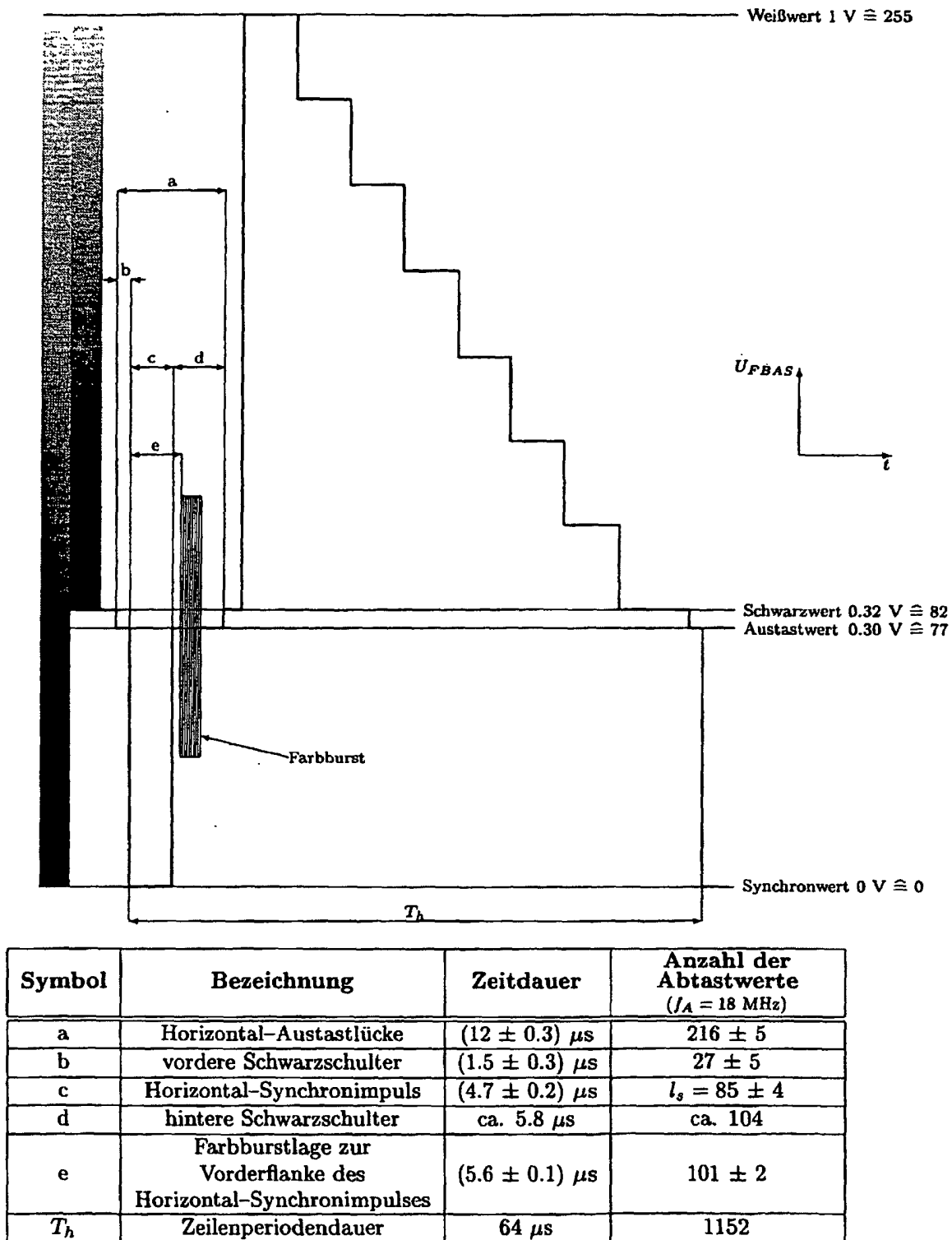
Fig. 3: Horizontal-Synchronsignal innerhalb einer Zeile (CCIR-Norm B,G)
