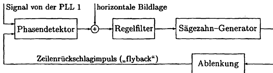
Fig. 10: Erzeugung des Steuersignals für die Horizontalablenkung (PLL 1)
