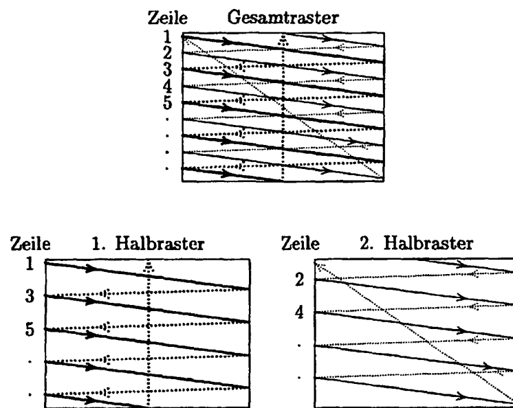
Fig. 2: Aufteilung des Gesamtrasters (vgl. Fig. 1) in zwei Halbraster beim Zeilensprungverfahren, punktierte Linien sind Strahlrückführungen
