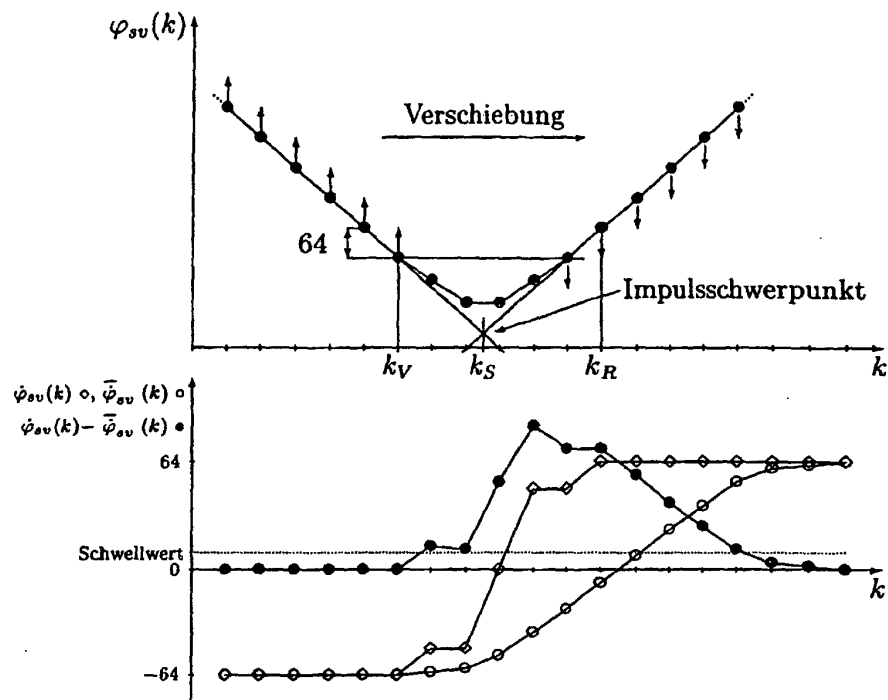
Fig. 14: Korrelationsfunktion \varphi_{sv}(k) des Impulses aus Fig. 13, ihre Ableitung \dot{\varphi}_{sv}(k) , ihre über m = 8 Werte gemittelte Ableitung \bar{\dot{\varphi}}_{sv}(k) und deren Differenz
