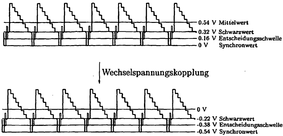
Fig. 8: Pegeländerung des FBAS-Signals bei Wechselspannungskopplung
