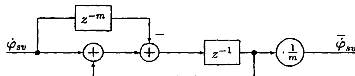
Fig. 16: Mittelung einer Abtastwertfolge über m Werte
