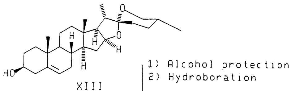
SCHEME VI
